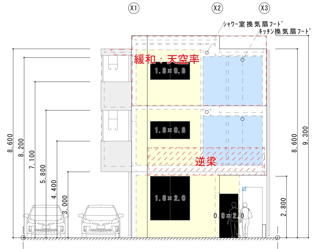
南側立面図
