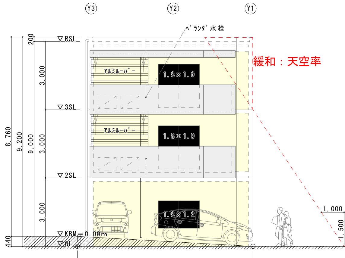
西側立面図
