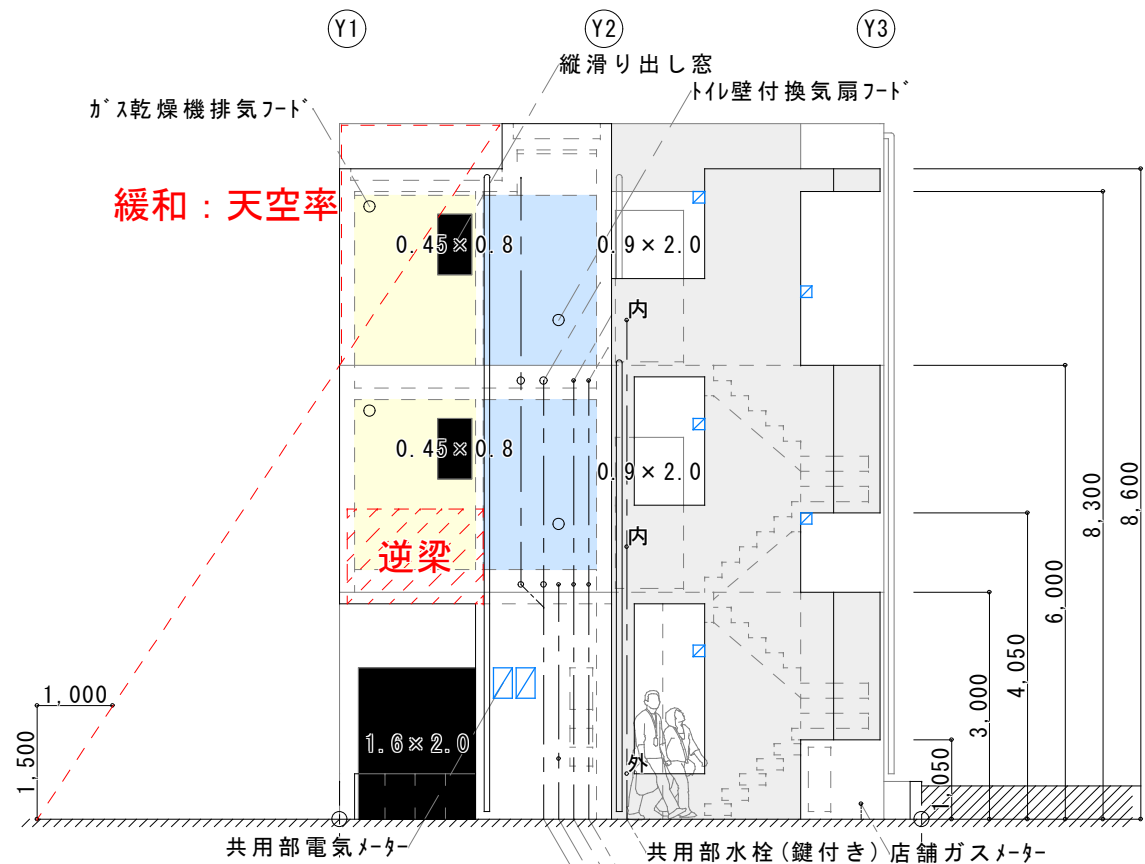
東側立面図
