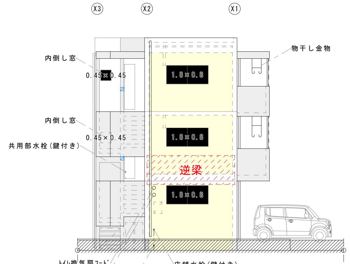
北側立面図
